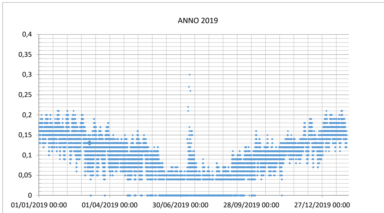
Grafico dell'Andamento nel tempo dei livelli medi orari dell'induzione magnetica, registrato dalla centralina di monitoraggio sita in via Colle Gesuiti 28 a Bucchianico.
