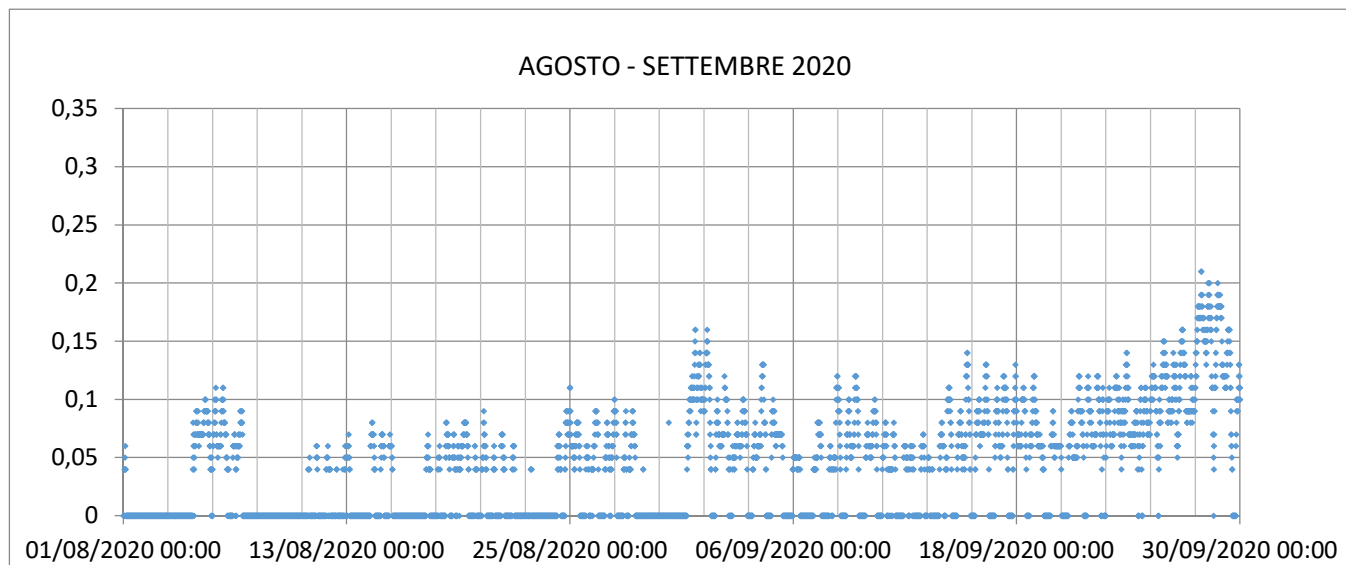
Grafico dell'Andamento nel tempo dei livelli medi orari dell'induzione magnetica, registrato dalla centralina di monitoraggio sita in Località Adriani - Casalincontro.
