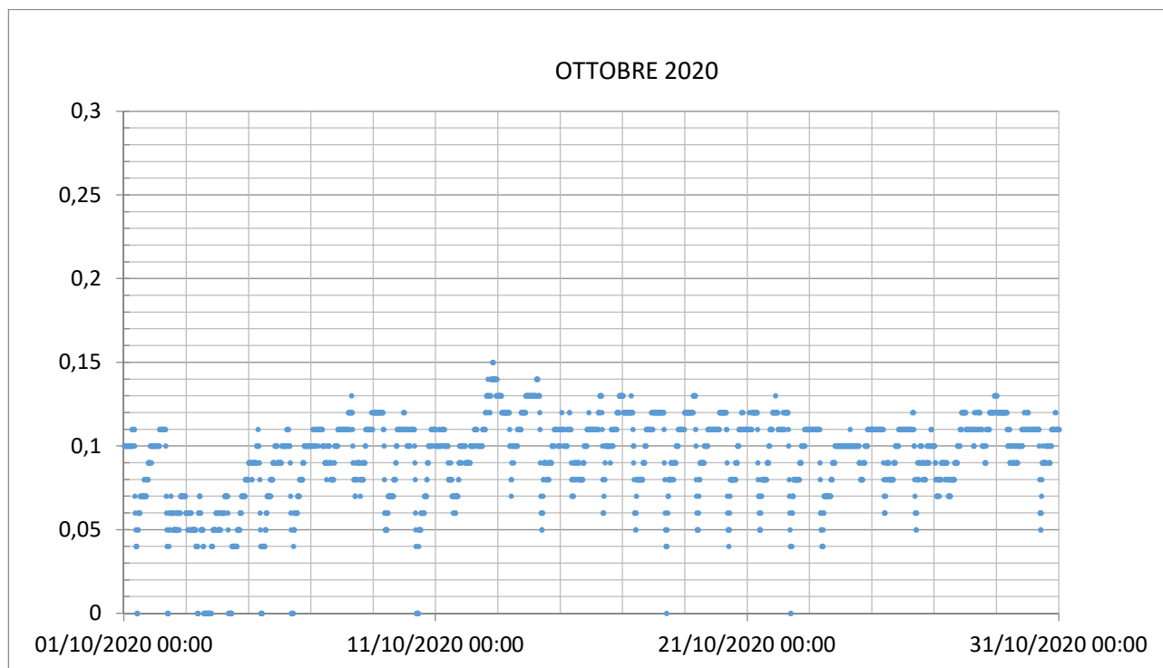
Grafico dell'Andamento nel tempo dei livelli medi orari dell'induzione magnetica, registrato dalla centralina di monitoraggio sita in C.da Sant'Onofrio a Lanciano.
